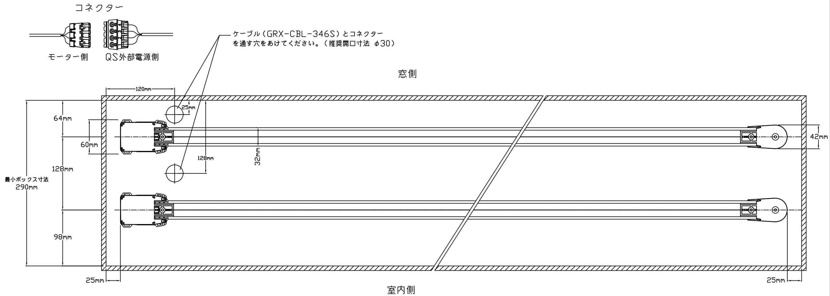
<上面図>
