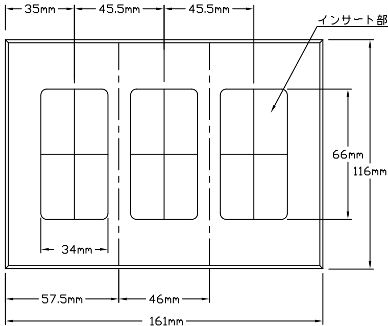
正面図
