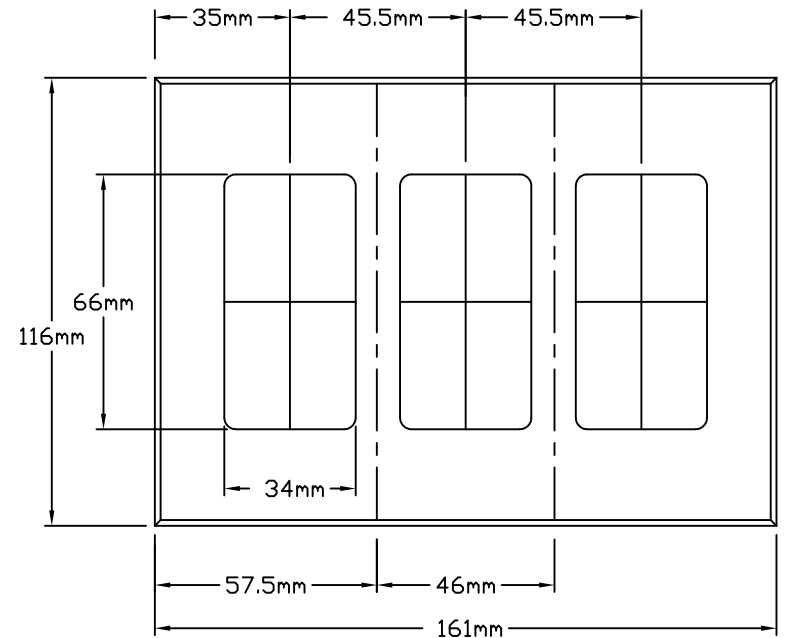
背面図
