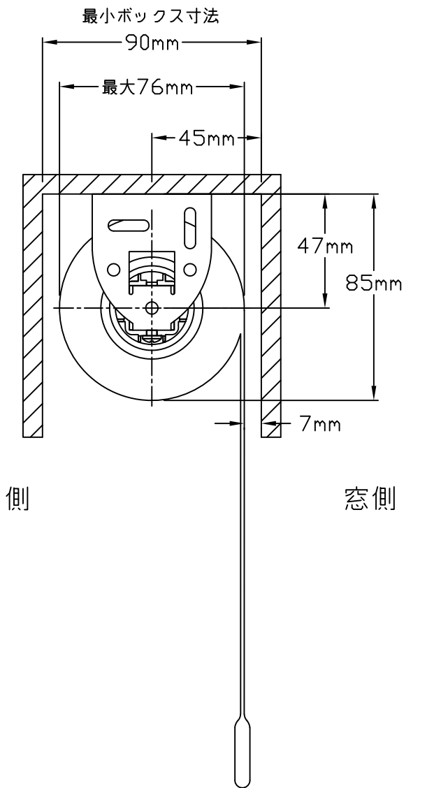
<側面図>
