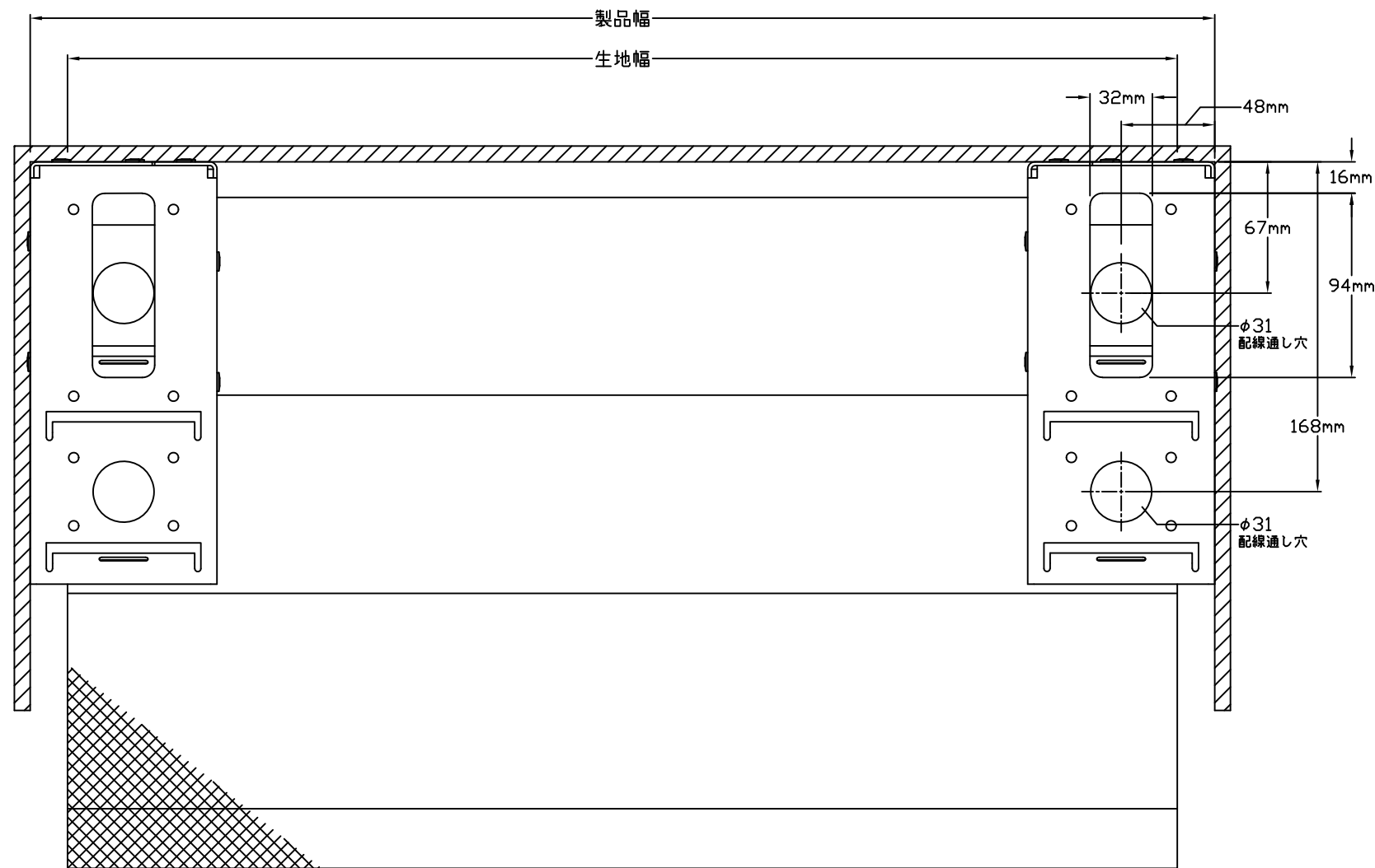
<正面図>
