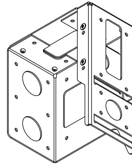
<右ブラケット 等角図>
