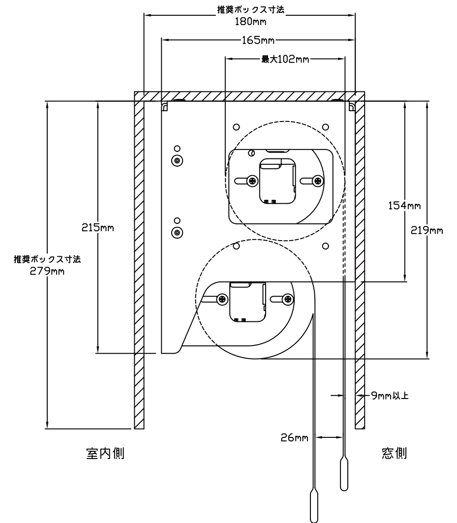
<側面図>
