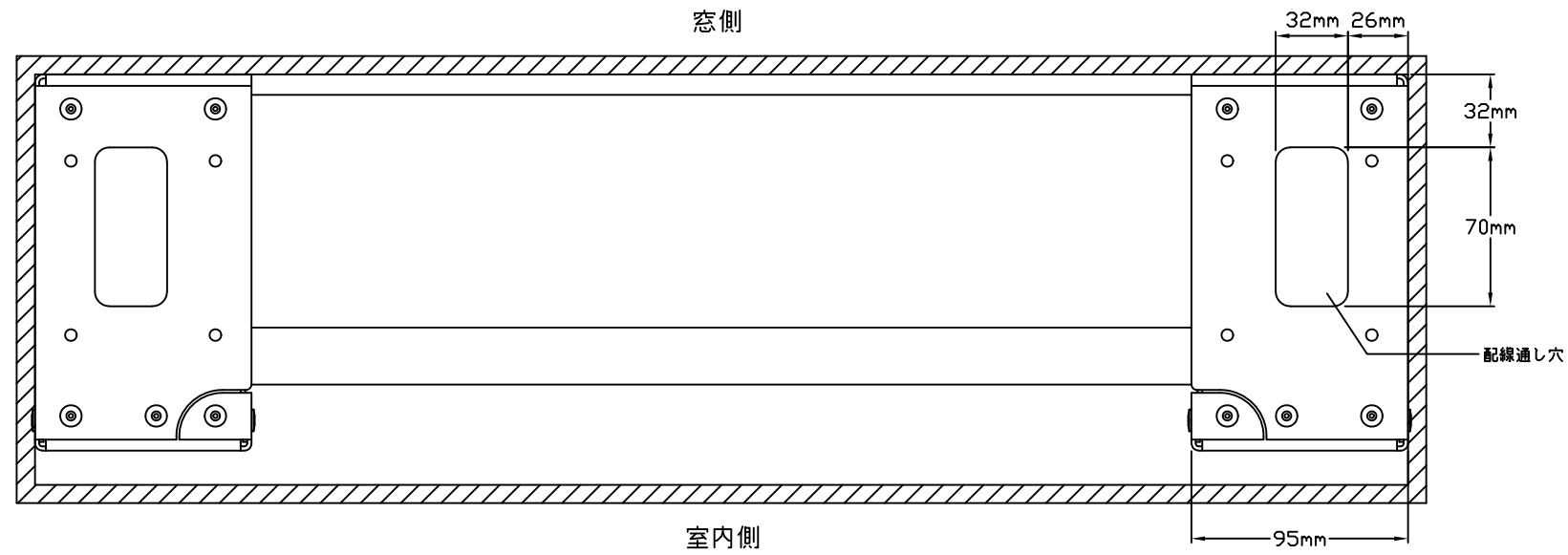
<上面図>
