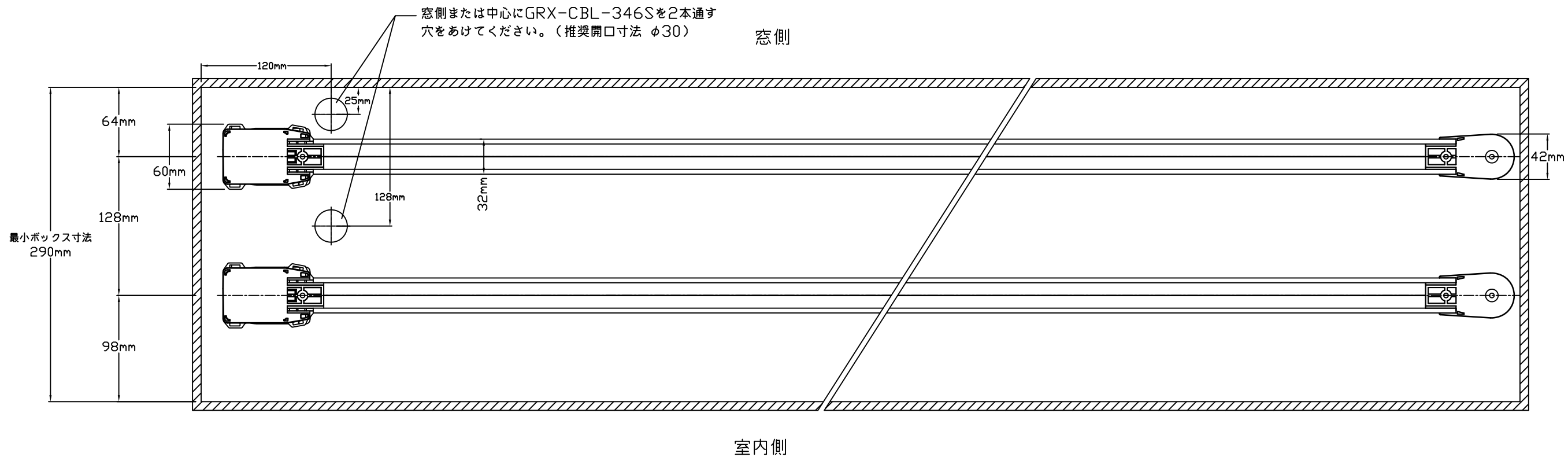
<上面図>
