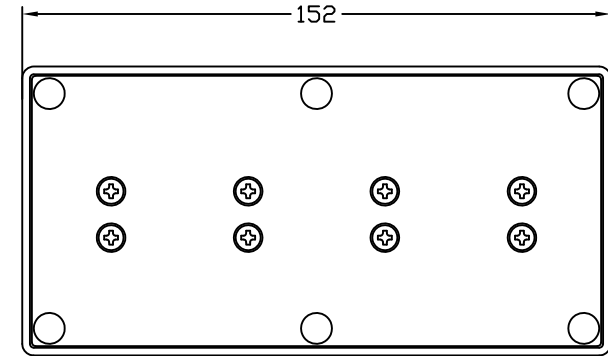
背面図
