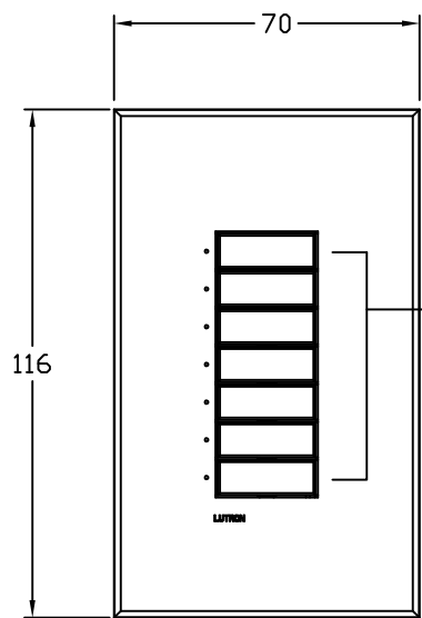
SQ-7BN / インサートなし 正面図 (フェースプレートを含む)
