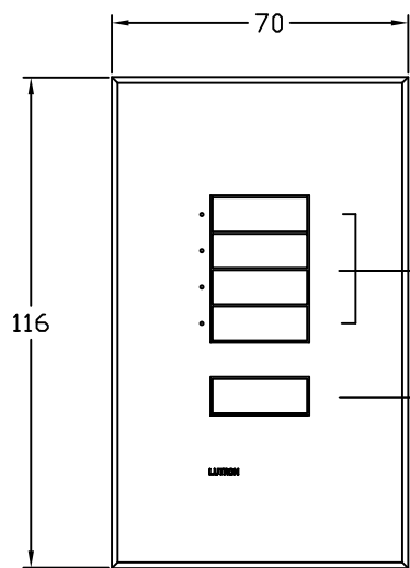
SG-4MN/インサートなし 正面図 (フェースプレートを含む)
