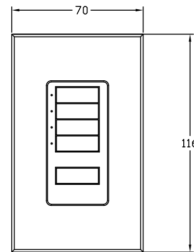
SG-4MI-/インサートあり 正面図 (フェースプレート含む)
