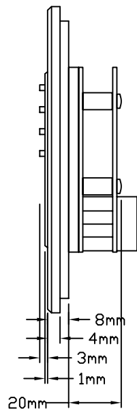
側面図 (フェースプレートを含む)
