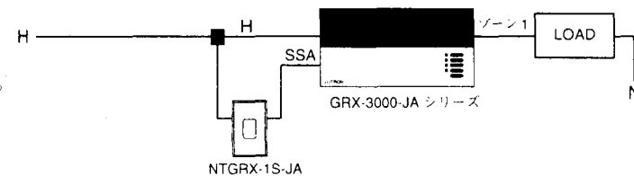
新たな取付け：GRX-3000-JAを電源側につなぐ場合
