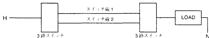
既存3路スイッチ配線図
