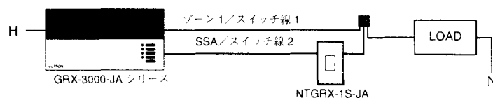
GRX-3000-JAを電源側に置いて既存配線を利用する場合
