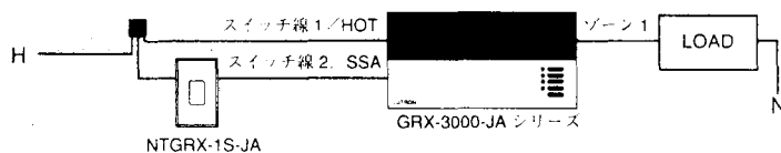
GRX-3000-JAを負荷側に置いて既存配線を利用する場合
