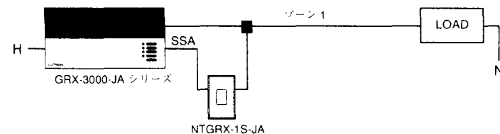
新たな取付け：GRX-3000-JAを負荷側につなぐ場合
