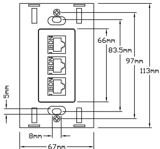
正面図 (フェースプレートを除く)
