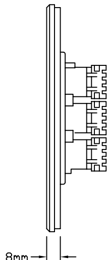
側面図 (フェースプレートを含む)
