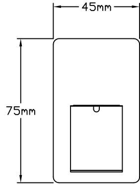
正面図(1個用)
