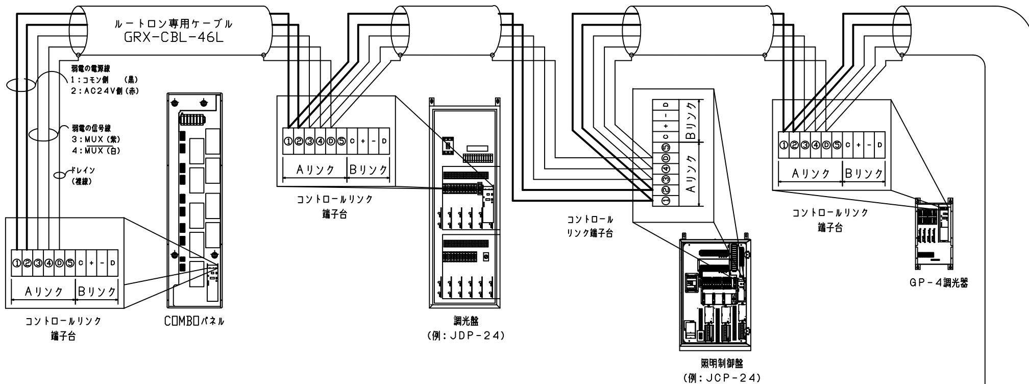
ルートロンケーブルGRX-CBL-346S/46L 色と端子
