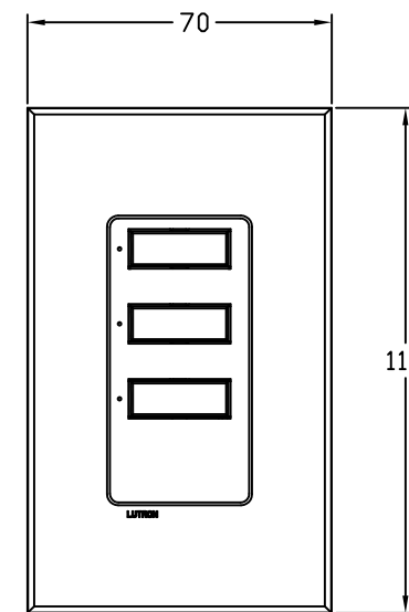
□-3BI / インサートあり 正面図 (フェースプレート含む)
