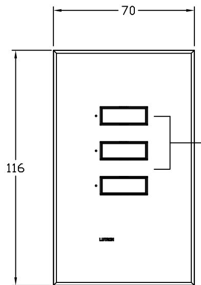
□-3BN / インサートなし 正面図 (フェースプレートを含む)
