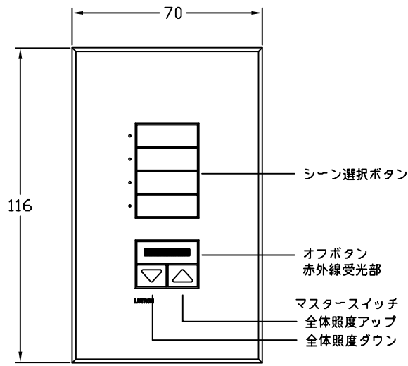
SG-4SIRN/インサートなし 正面図 (フェースプレートを含む)
