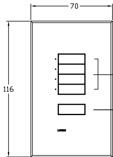
SG-4MN/インサートなし 正面図 (フェースプレートを含む)
