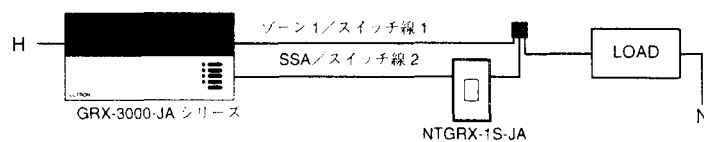
図1 既存配線を利用する場合
