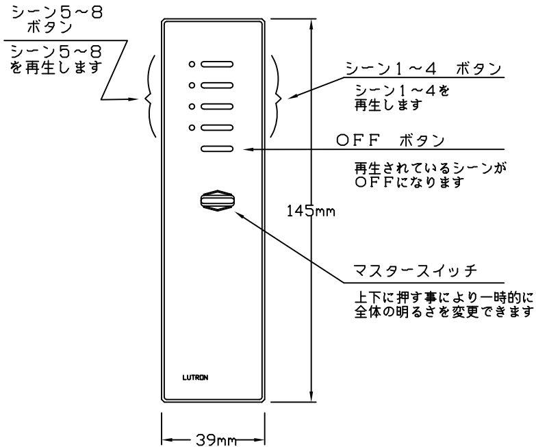
正面図
